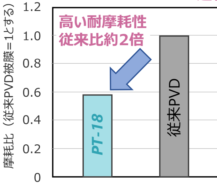
Fig. 実機耐久後被膜摩耗比および摺動面状況
